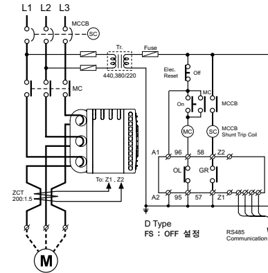
3상 모터 결선도 (MCCB 차단 예)
