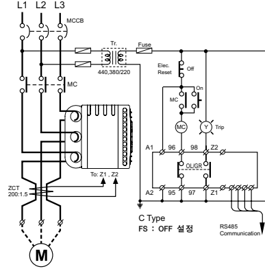
3상 모터 결선도 (출력접점 "C" Type, 공통접점)
