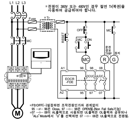
모터보호용 EOCR-FDE 3선 결선도 (FS : oFF설정)
